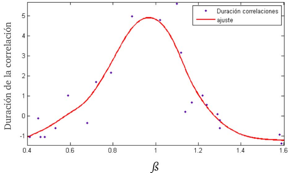
Figura 27. Ajuste aproximado de la correlación en cada hashtag respecto a su factor \beta . Los hashtags con un factor \beta cercano a 1 tienen más probabilidad de mantener su identidad durante más tiempo.
