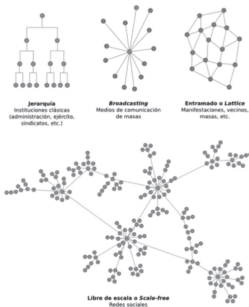
Figura 31. Arriba: tipos de topología de las formas de organización y comunicación social previas a internet y las tecnologías móviles. Abajo: topología de una pequeña red libre de escala generada mediante el modelo de Barabási-Albert. Hay unos pocos nodos con muchas conexiones y muchos nodos con pocas conexiones de acuerdo a una distribución libre de escala.
