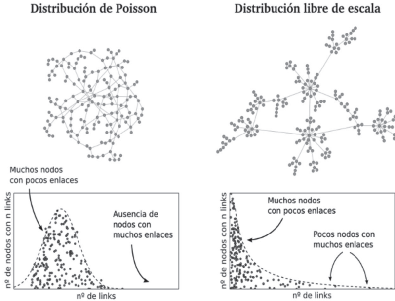
Figura 30. Distribución normal (límite de Poisson) generada mediante el modelo Erdos-Renyi y distribución libre de escala generada mediante el modelo Barabási-Albert. Ambas redes cuentan aproximadamente con 200 nodos y 200 enlaces.
