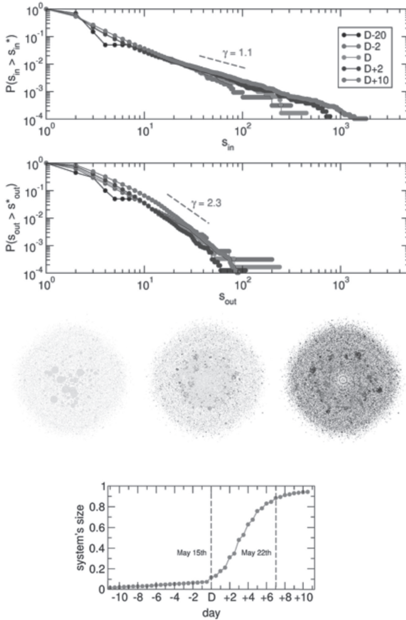
Figura 32. Arriba: Estructura libre de escala en la conectividad efectiva de las redes de comunicación del 15M en Twitter. Abajo: transición de fase (o percolación) en la conectividad y crecimiento de las redes de Twitter del 15M. Figura tomada de (Borge-Holthoefer et al., 2011) con licencia CC-by.
