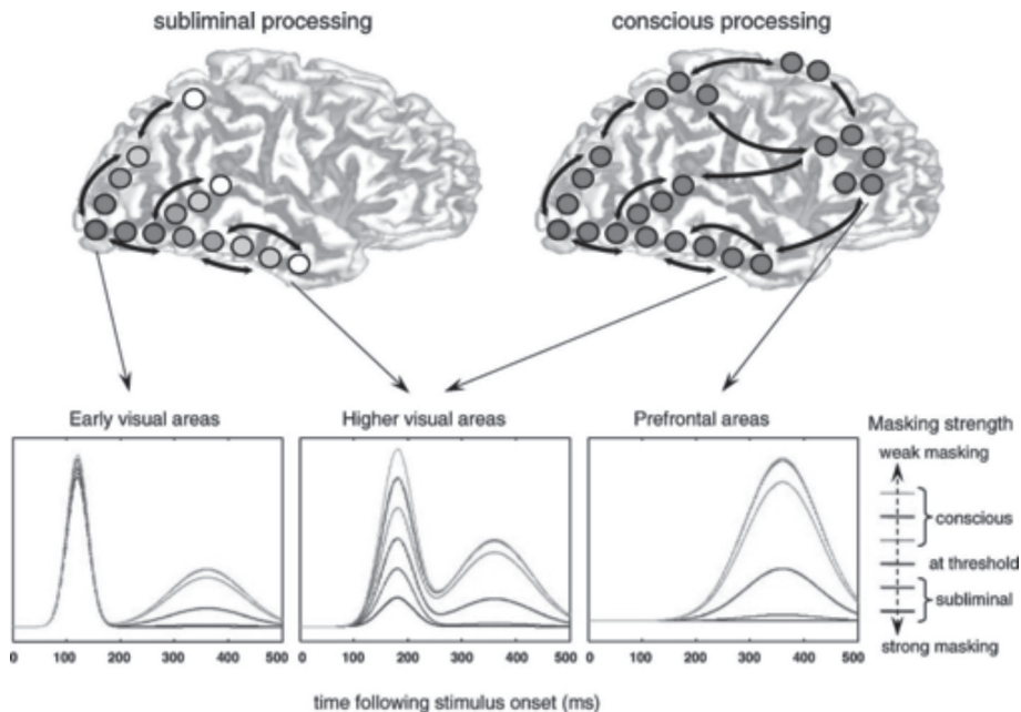
Figura 34. Ilustración del devenir consciente de un estímulo visual. Los estímulos que se presentan por tiempo corto no llegan a extender su influencia al resto del cerebro (especialmente a las áreas prefrontales). Véase figura 35 para una explicación más detallada. Tomado de Del Cul, Baillet y Dehaene (2007) con licencia CC-by.
